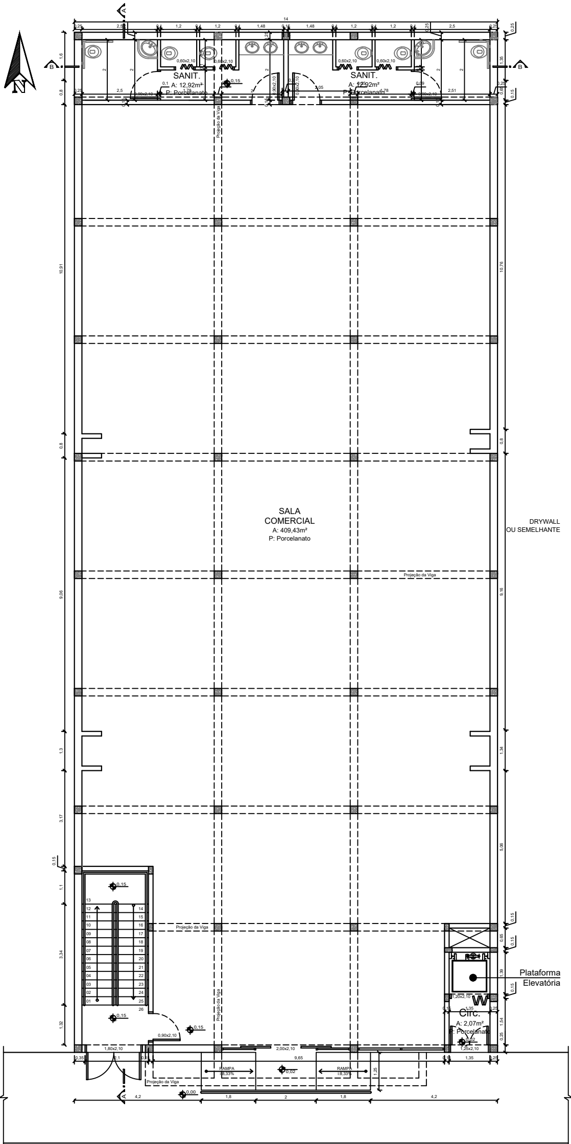
PLANTA BAIXA TÉRREO A: 473,90m 2 Esc: 1/75
